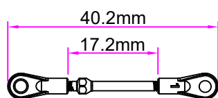
M1.6 舵机连杆 (Servo Linkage Rod)
